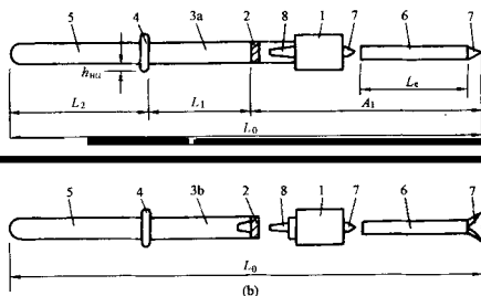
图 1 验电器
