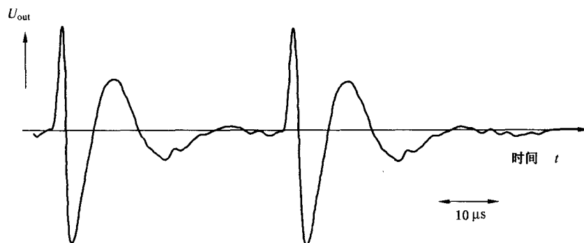
图 E1. b 带宽 \Delta f = 45 \text{ kHz} \sim 440 \text{ kHz} , 长时输入脉冲
